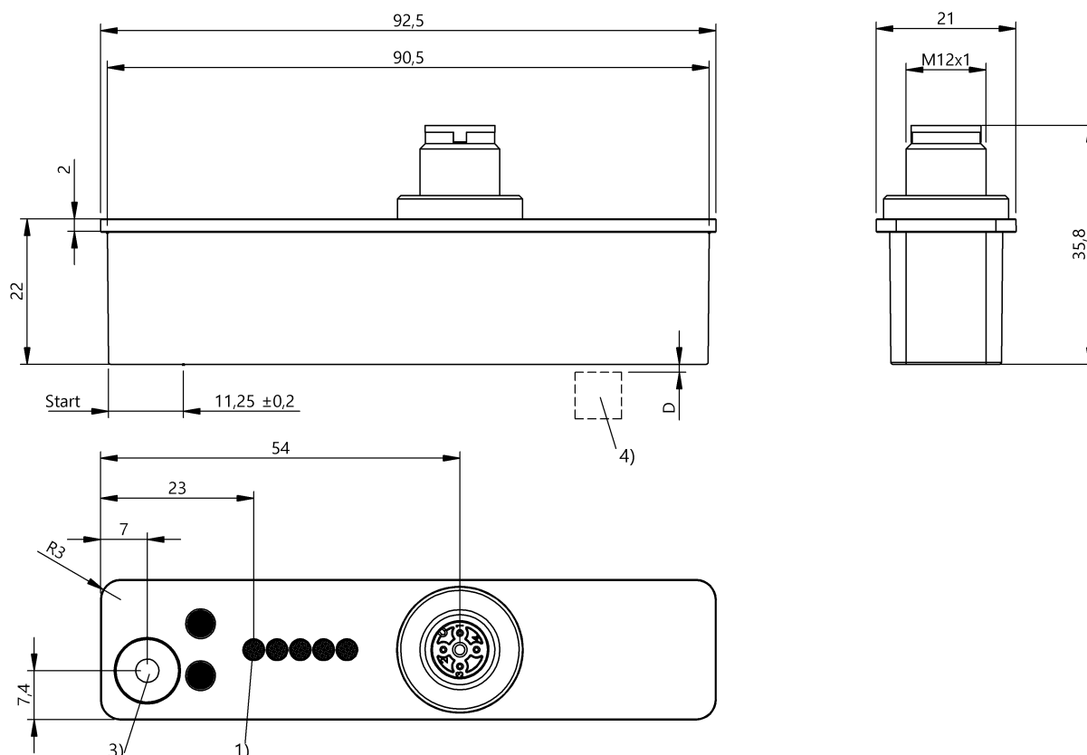
1) Функциональный СД, 3) Кнопка запоминания, 4) Датчик положения
